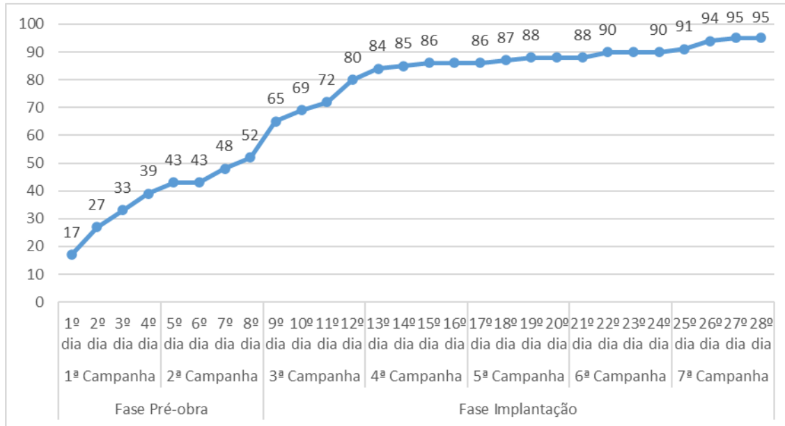
Figura 53 - Gráfico com curva de acúmulo de espécies com base nos dados levantados durante as campanhas de monitoramento de fauna para a CGH Teles de Proença.
