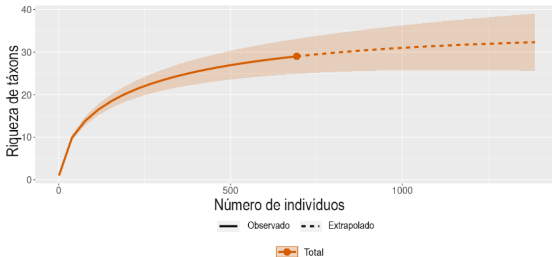
Figura 20 - Gráfico de curva de rarefação de macroinvertebrados aquáticos coletado nas seis campanhas para CGH Teles de Proença.
