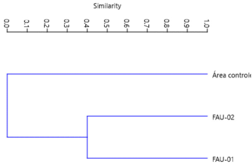
Figura 79 - Dendrograma de Similaridade de Jaccard para as áreas da CGH Teles de Proença durante a sétima campanha.
