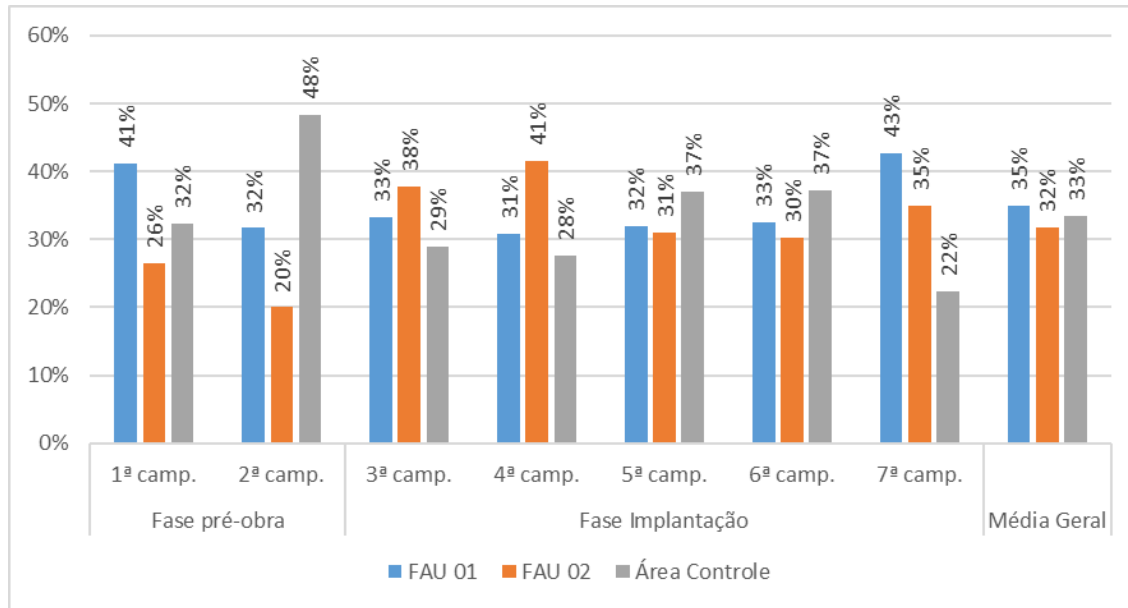
Figura 51 - Gráfico de riqueza de espécies para os três pontos de monitoramento de fauna, nas sete campanhas da CGH Teles de Proença.
