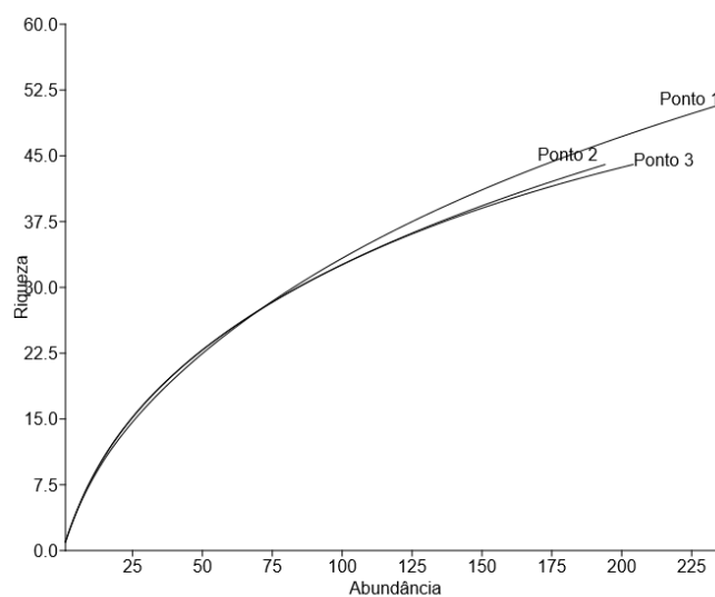
Figura 12 - Gráfico comparativo pelo método de rarefação da assembleia de insetos amostrados em três pontos na área de influência direta da CGH Teles de Proença.
